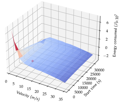
(d) Energy graph for segment 3.
