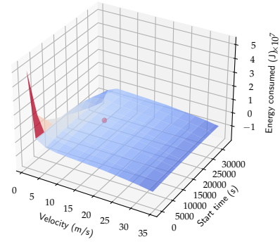
(d) Energy graph for segment 348.
