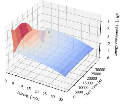
(d) Energy graph for segment 66.
