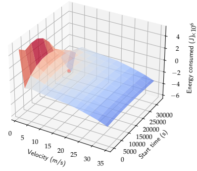
(d) Energy graph for segment 60.
