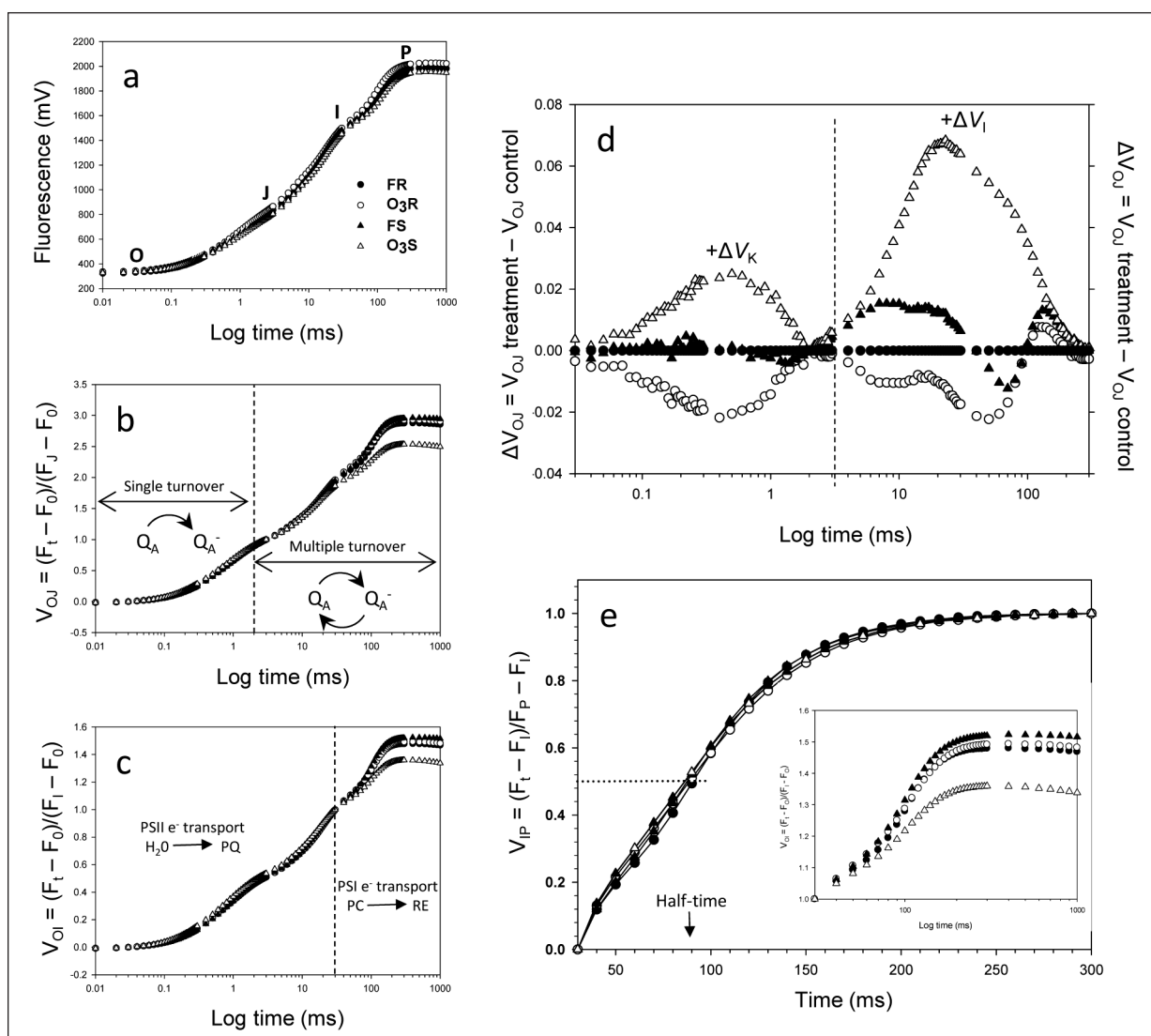
FIGUUR 2: Vinnige fase chlorofil \alpha -fluoressensiekinetika van intakte blare van die verskillende behandelings en genotipes na 25 dae se blootstelling aan 80 nmol. mol -1 O_3 . (a): Gemiddelde onverwerkte fluoressensiekrommes vóór aanvang van O_3 -blootstelling; (b): Gemiddelde fluoressensiekrommes, dubbeld genormaliseer tussen F_0 (50 s en F_J (2 ms) op logaritmiëse tydskaal, wat die relatiewe verandering in die enkel-omsettingsfase (0 – 2 ms) en die meervoudige omsettingsfase (2ms – ~ 300 ms) aantoon; (c): Gemiddelde fluoressensiekrommes dubbeld genormaliseer tussen F_0 (50 \mu s) en F_P (30 ms) op logaritmiëse tydskaal, wat die relatiewe verandering in die enkel-omsettingsfase (0 – 2 ms) en die meervoudige omsettingsfase (2ms – ~ 300 ms) aantoon; (d): Verskil in varieerbare fluoressensie ( \Delta V = V_{\text{behandeling}} - V_{\text{kontrolle}} ) teenoor log-tyd van die verskillende behandelings en genotipes genormaliseer tussen die fluoressensie-ekstreem F_0 (50 \mu s) en F_J (2 ms), en F_J (2 ms) en F_P onderskeidelik, om die \Delta V_{OJ} en \Delta V_{JP} krommes te verkry wat die \Delta V_K en \Delta V_I bande blootlê; (e), inset: Gemiddelde fluoressensiekrommes genormaliseer tussen F_0 (50 \mu s) en F_P (30 ms) wat die V_{OI} -gedeelte vir waardes groter as 1 (na 30 ms) oor die tydverloop 30 -300 ms aantoon. Die I-P-styging weerspieël die grootte van die pool van eidelektronontvangers; (e), hoofgrafiek: Gemiddelde fluoressensiekrommes van behandelings en genotipes, onderskeidelik genormaliseer tussen F_J (30 ms) en F_M (piek) en voorgestel op 'n lineêre skaal tussen 30 – 300 ms met die maksimumamplitude vasgestel op 1 ten einde die reduksietempo van eidelektronontvangers van die verskillende behandelings te vergelyk. FR is as verwysing/kontrolle gebruik. Elke kromme verteenwoordig die gemiddelde van 48 metings.
