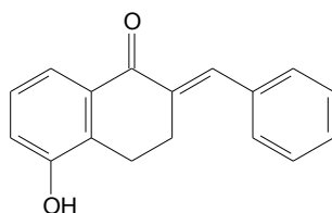
( E )-2-Benzylidene-5-hydroxy-1-tetralone
