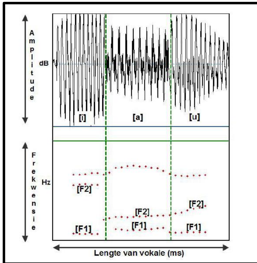
Figuur 4.1: Ossillogram van [i, a, u] wat ook formante F1 en F2 wat daarmee geassosieer word, aandui (geneem uit Wissing, 2014a:108)
