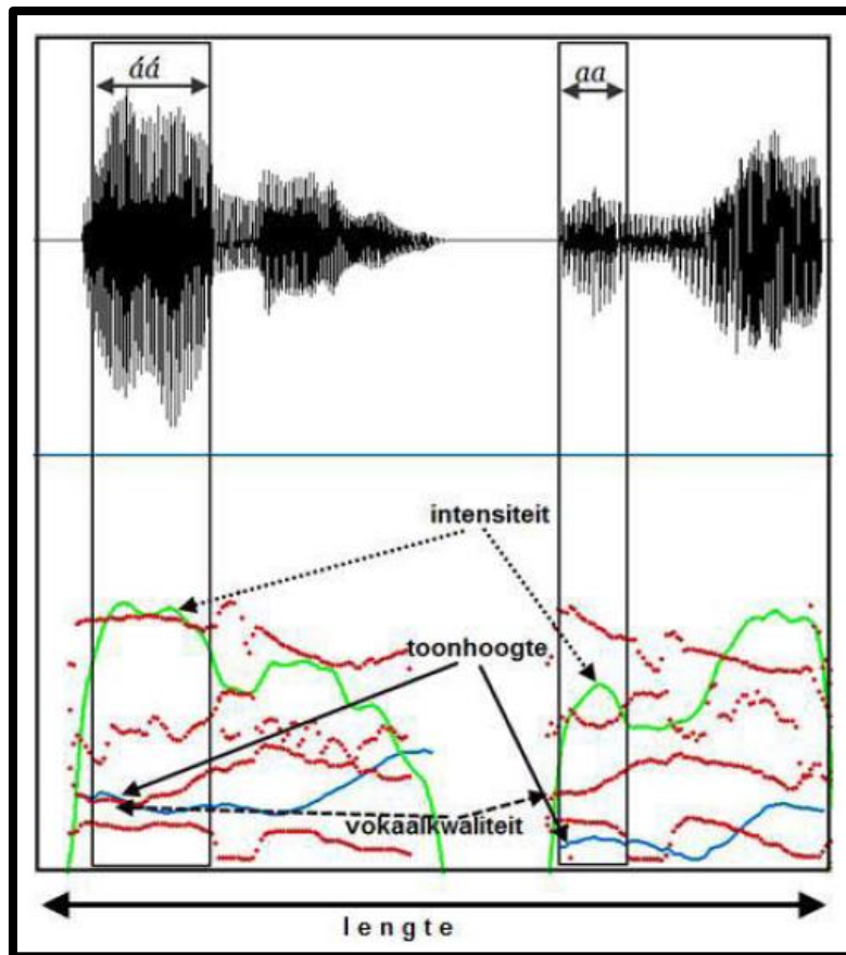
Figuur 4.2: Ossillogram (bo) van áánhou- en aanhóú- in die woord. Onder word intensiteit, grondtoon en formantfrekwensies aangedui (geneem uit Wissing, 2014b:158).
