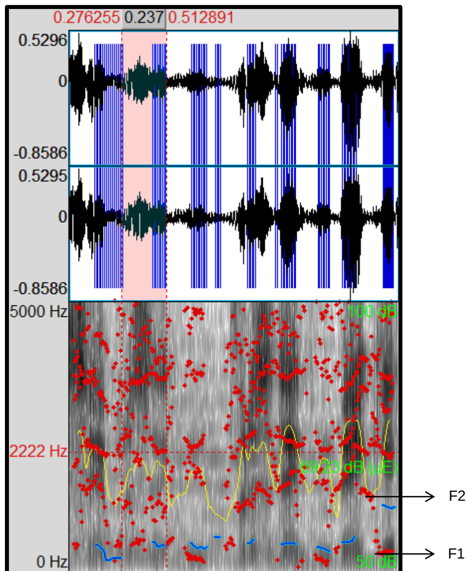
Figuur 4.13: Akoestiese analise van 'n vals inleiding soos by [8:2]
