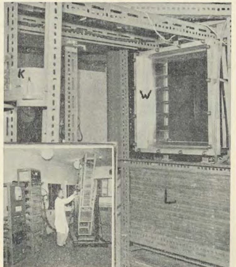
Die Wilson-Wolkekamer waarmee die direkte paarvorming van /u-mesone ondersoek word. W = wolkekamer, K = outomatiese kamera, L = 35 cms. loodplate.
